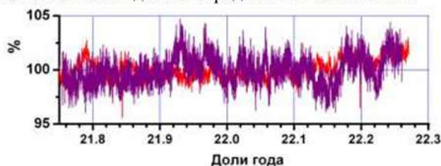
Рисунок 3. Вариации отношения счета НМ (НМ_Ап)/(НМ_Бр), красный цвет, и отношения счета МТ (МТ_Ап)/(МТ_Бр), лиловый цвет.
